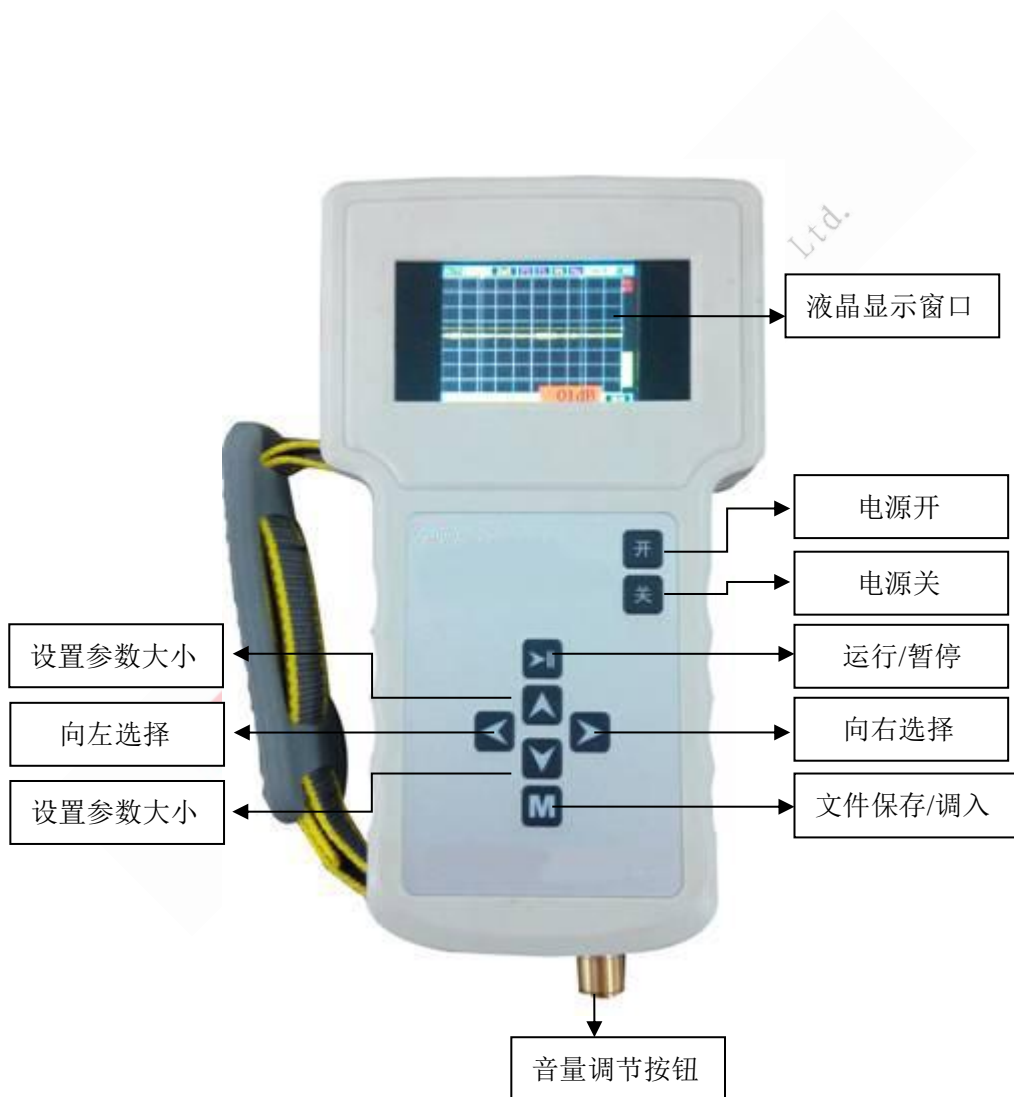
主机正面图
