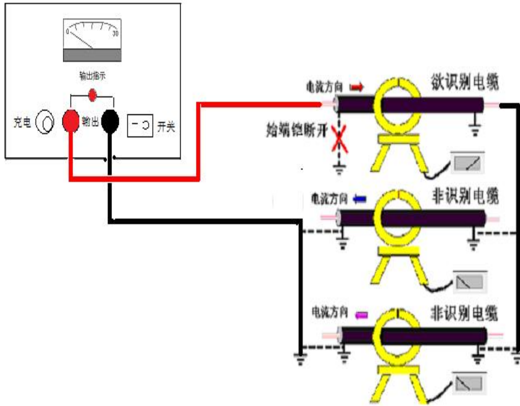
测试步骤三 不带电电缆识别工作判别
