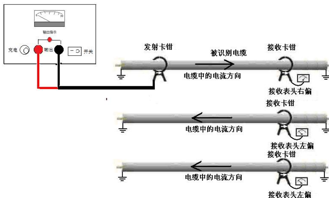
带电电缆识别工作判别
