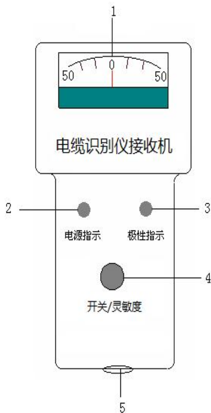
图 3-2 电缆识别仪接收机面板图
