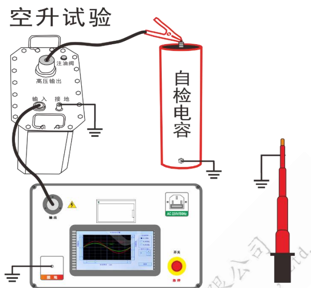
图 17 仪器空升自检接线示意图
