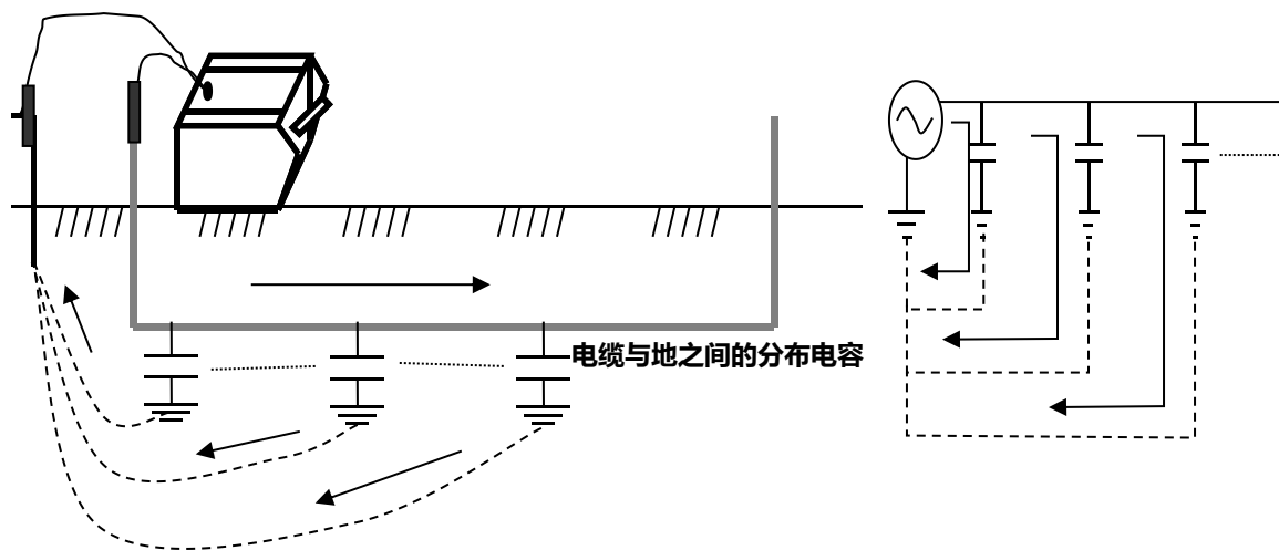
直连法容性回路(终端未接地) — 示意图
