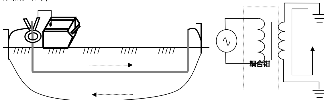
耦合法接线—示意图
