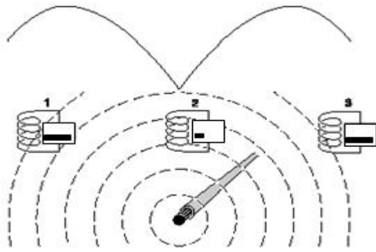
波谷法原理图
