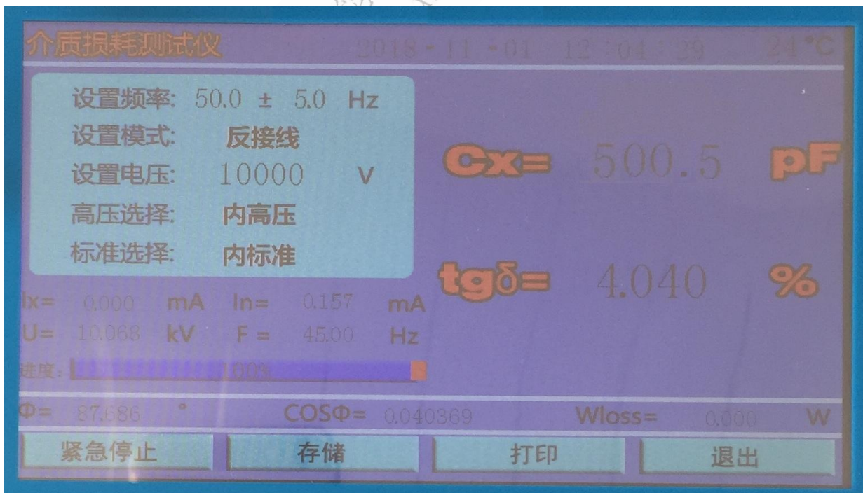
图十 反接线测试结果
