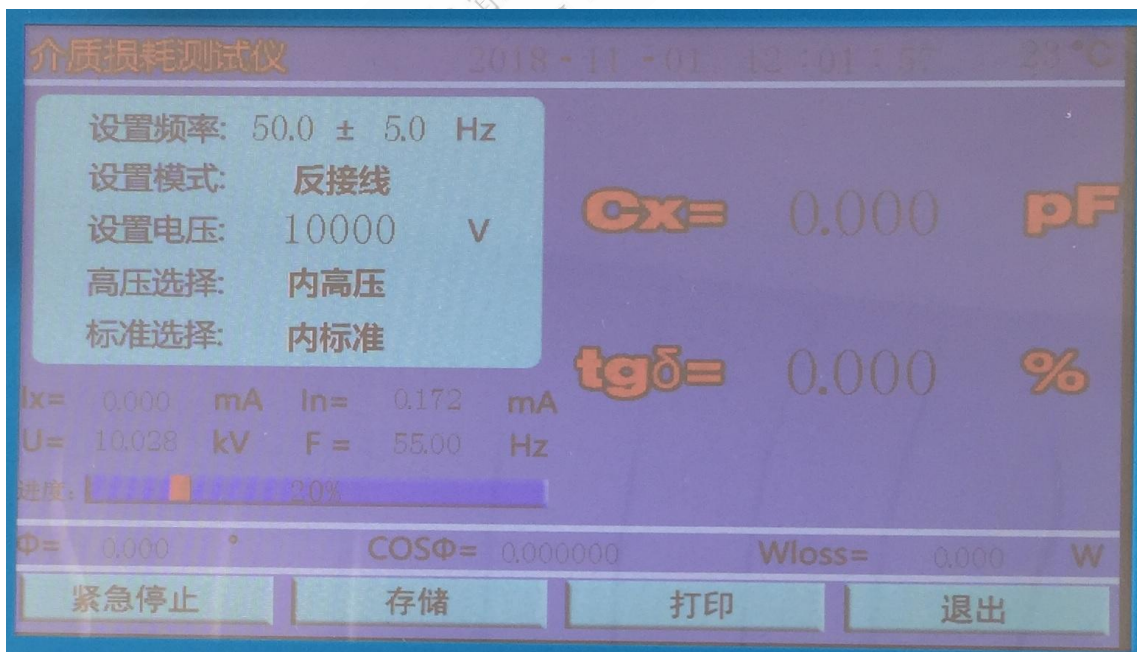
图八 仪器 55Hz 测试
