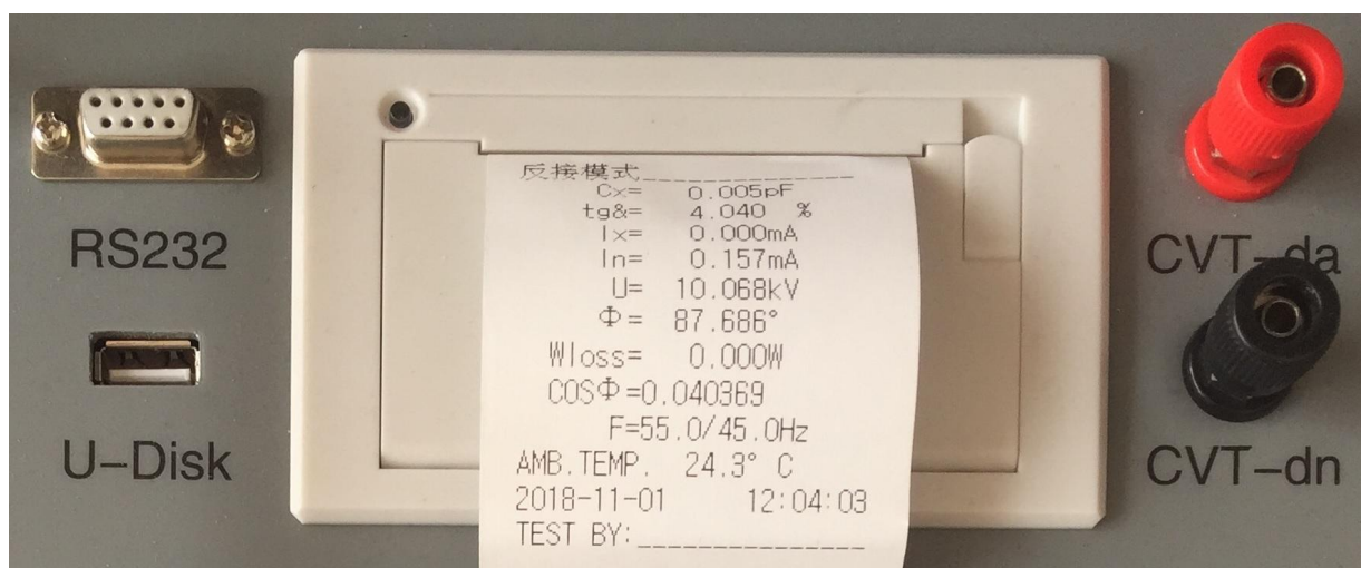
图十五 数据打印图
