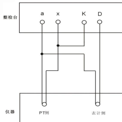
PT 二次压降检定接线图
