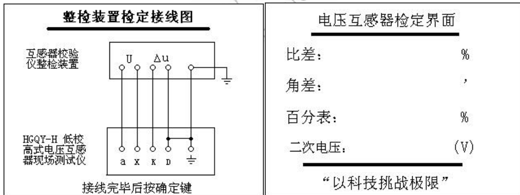
图 6-10 整检装置检定接线图
