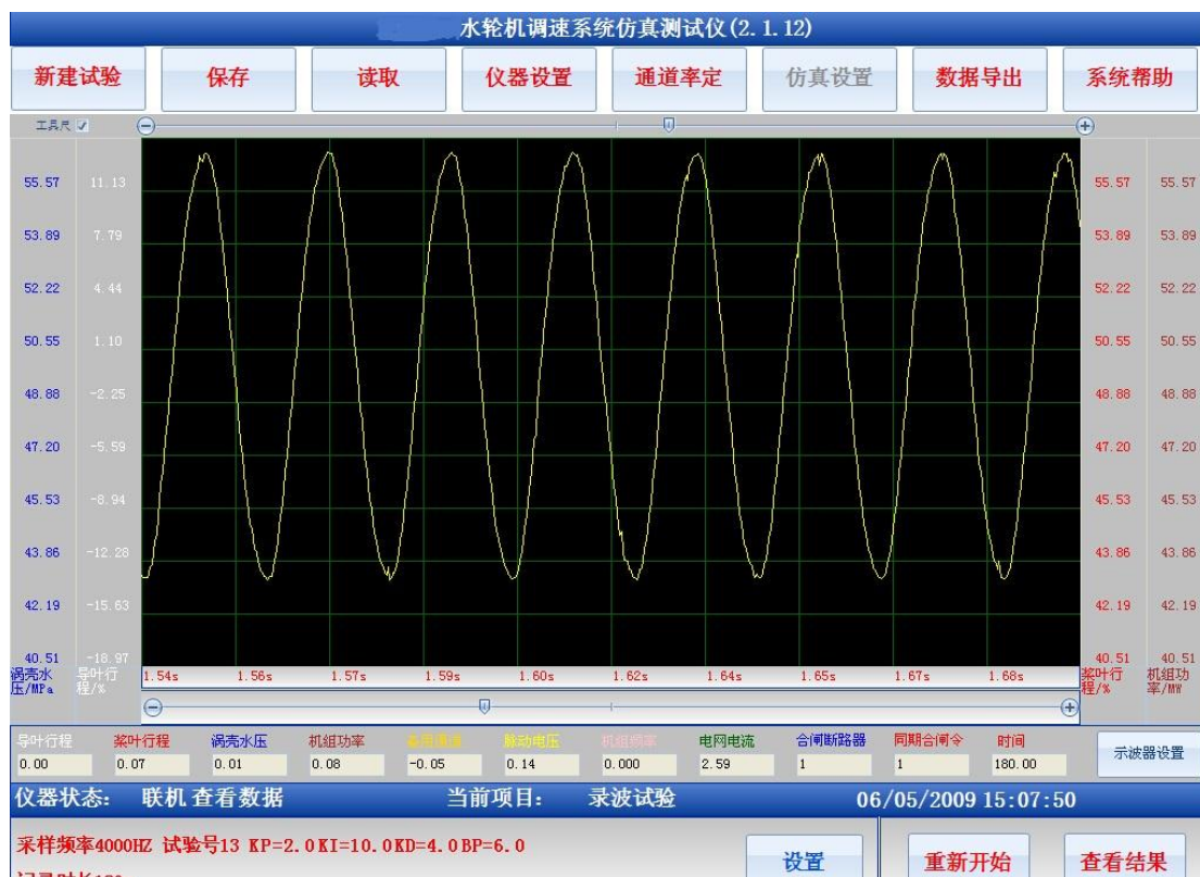
图 4.8 录波曲线
