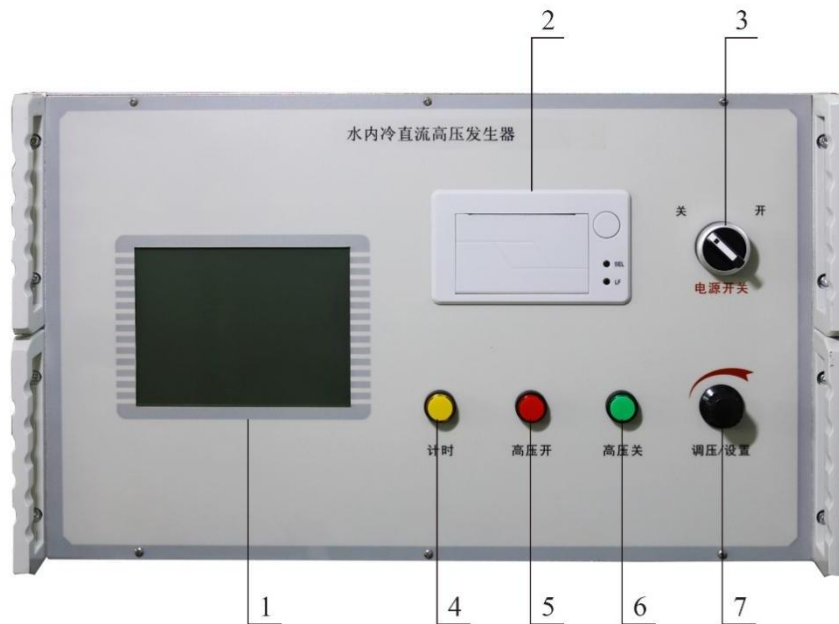
图 4-1 面板
