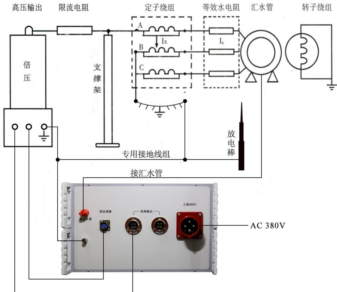
图六 试验回路接线图
