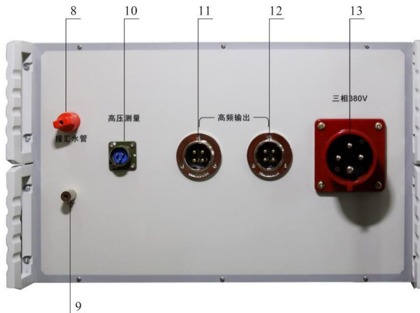
图 4-2 背板
