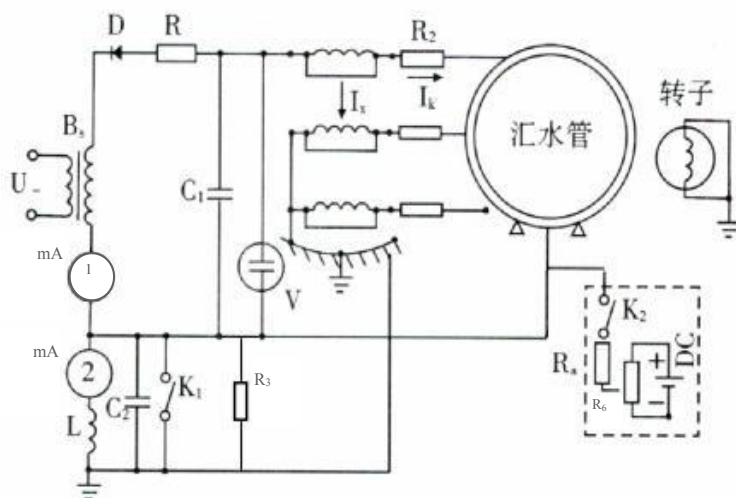
图 1 直流试验低压屏蔽法接线
