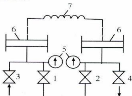
图 2 “充水”示意图
